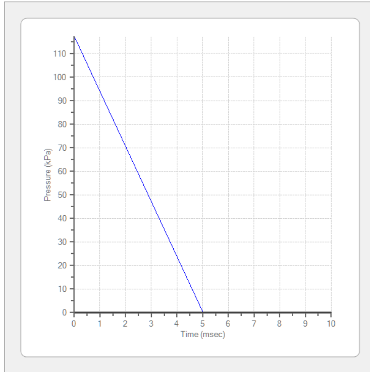
Blast Load
